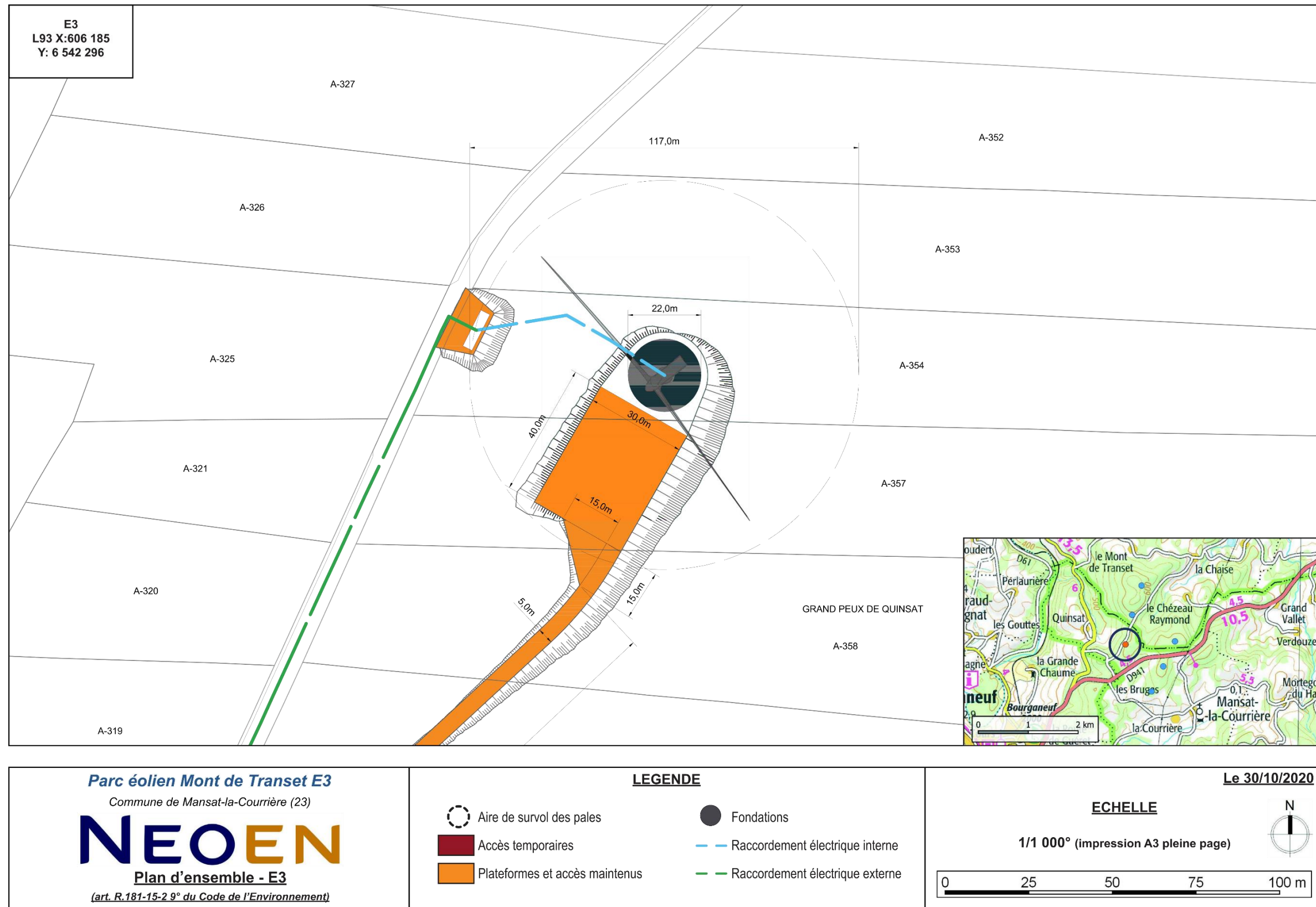
Carte 13 : Plan de masse du parc éolien du Mont de Transet – E3 (1/2)
