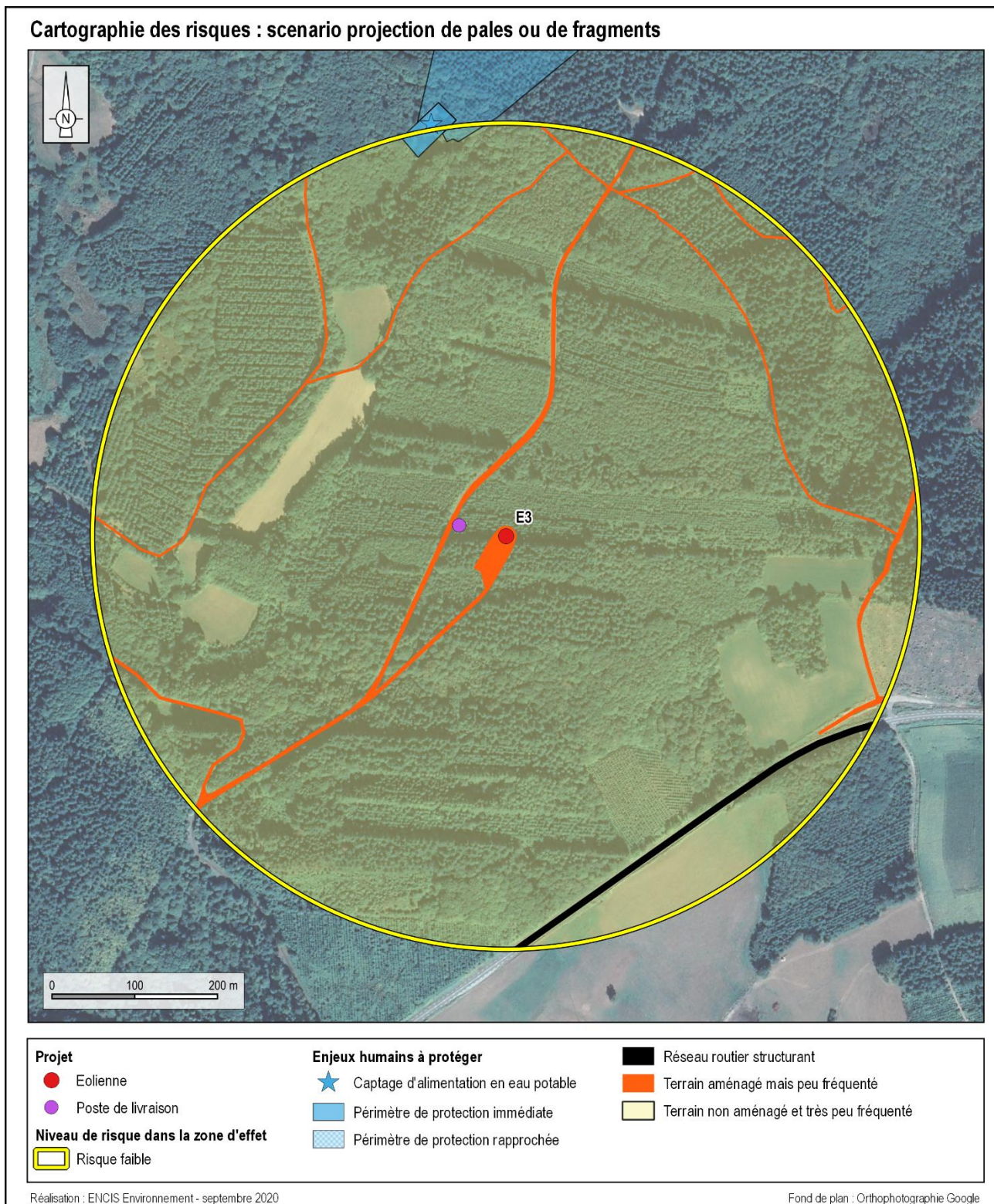
Carte 12 : Cartographie des risques – Scénario de projection de pales ou de fragments de pales
