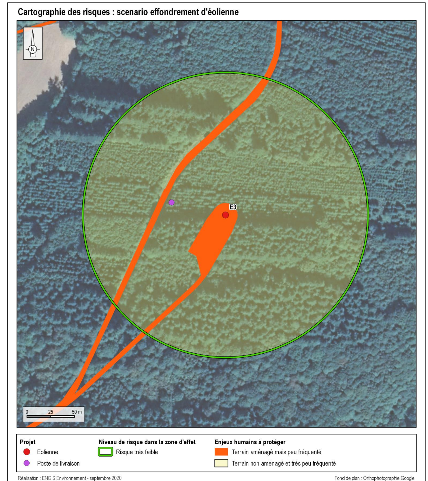
Carte 9 : Cartographie des risques – Scénario d'effondrement de l'éolienne
