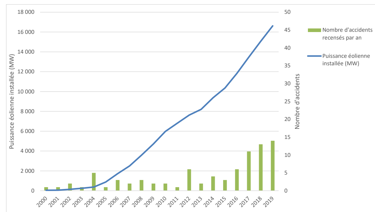
Figure 11 ; Evolution du nombre d'accidents annuels en France et puissance éolienne installée depuis 2000
