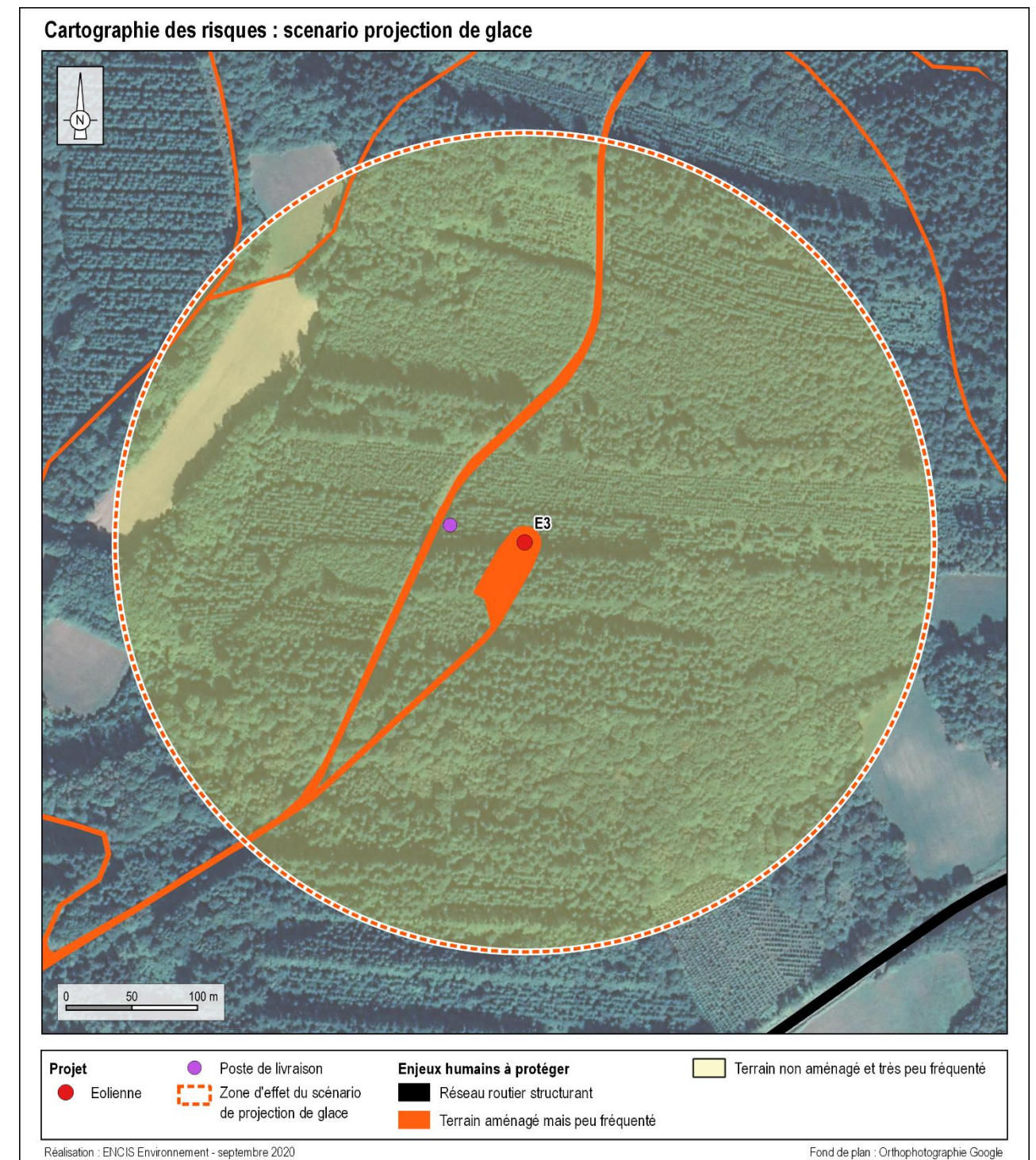
Carte 19 : Cartographie des enjeux identifiés dans la zone d'effet du scénario de projection de glace
