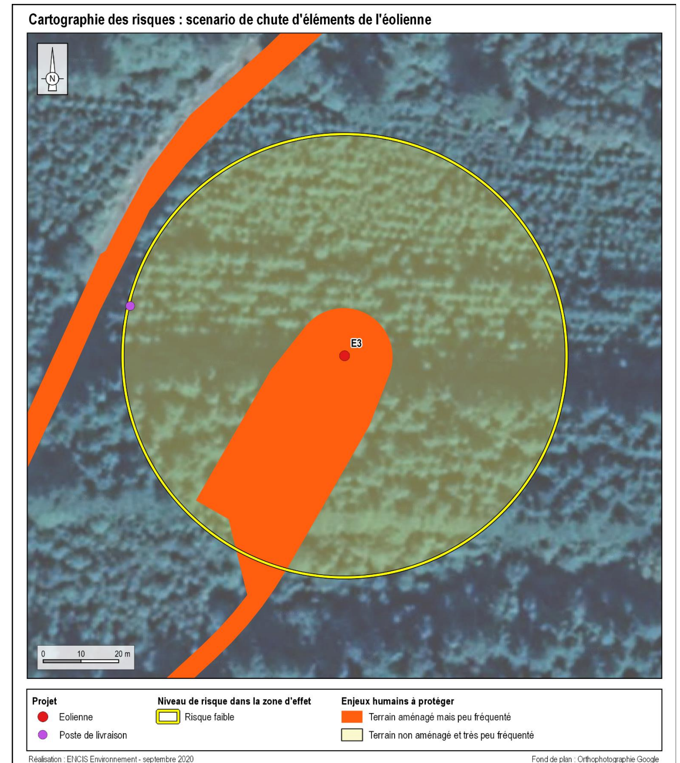
Carte 11 : Cartographie des risques – Scénario de chute d'éléments de l'éolienne
