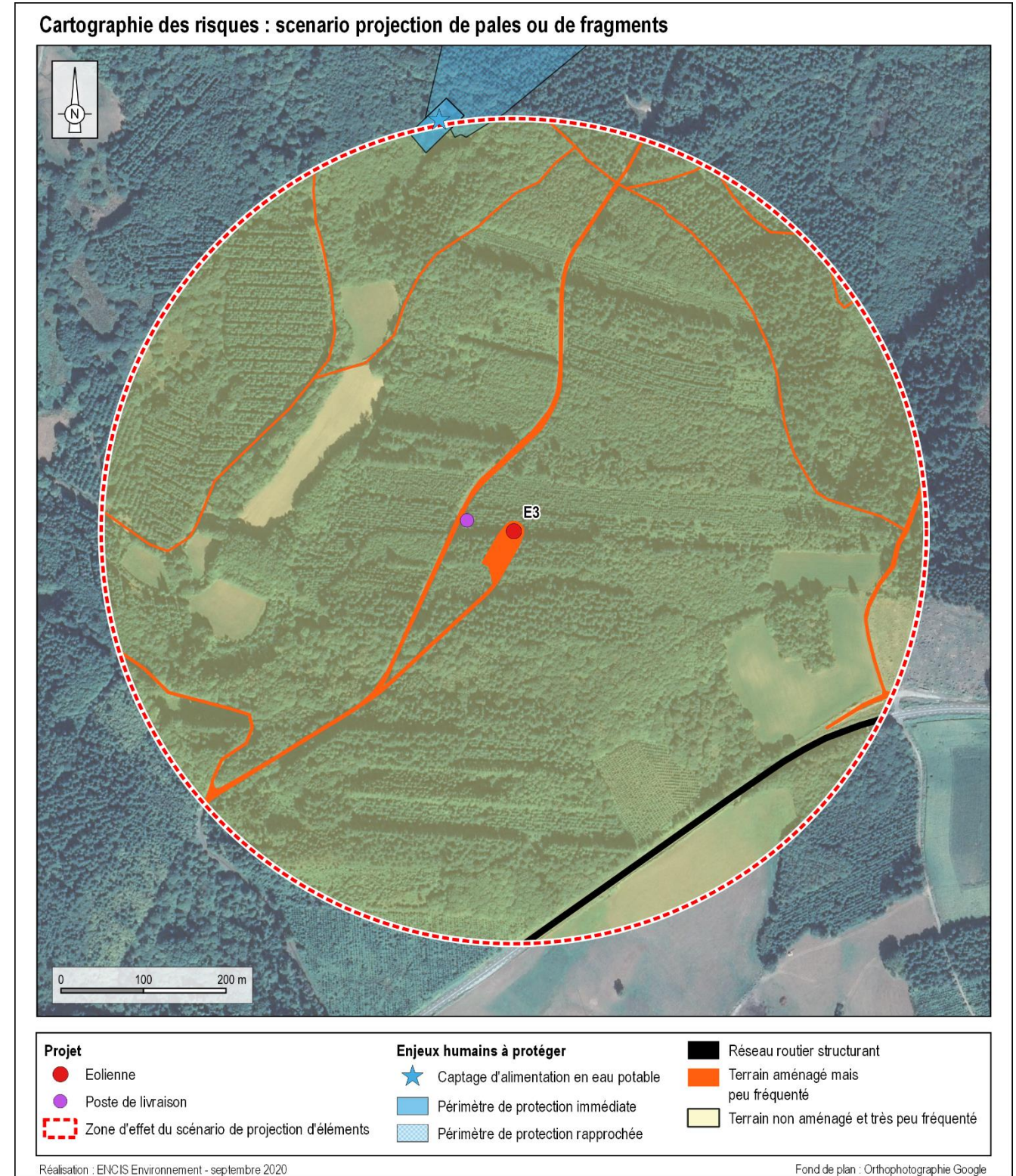
Carte 18 : Cartographie des enjeux identifiés dans la zone d’effet du scénario de projection de pales ou de fragments de pales
