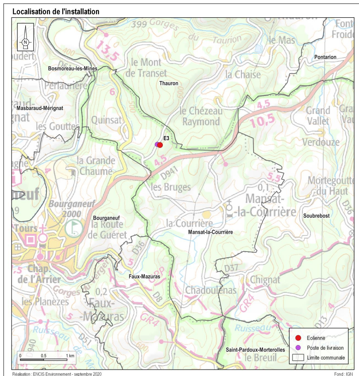
Carte 2 : Localisation de l'éolienne du parc éolien du Mont de Transet - E3
