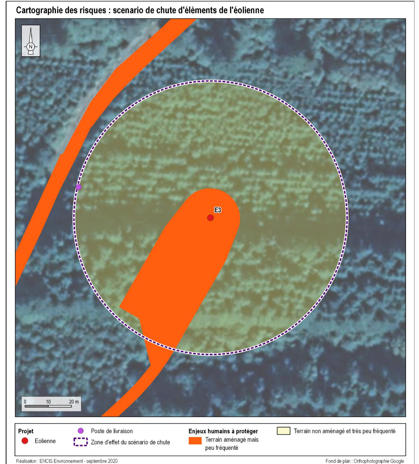
Carte 17 : Cartographie des enjeux identifiés dans la zone d'effet du scénario de chute d'éléments
