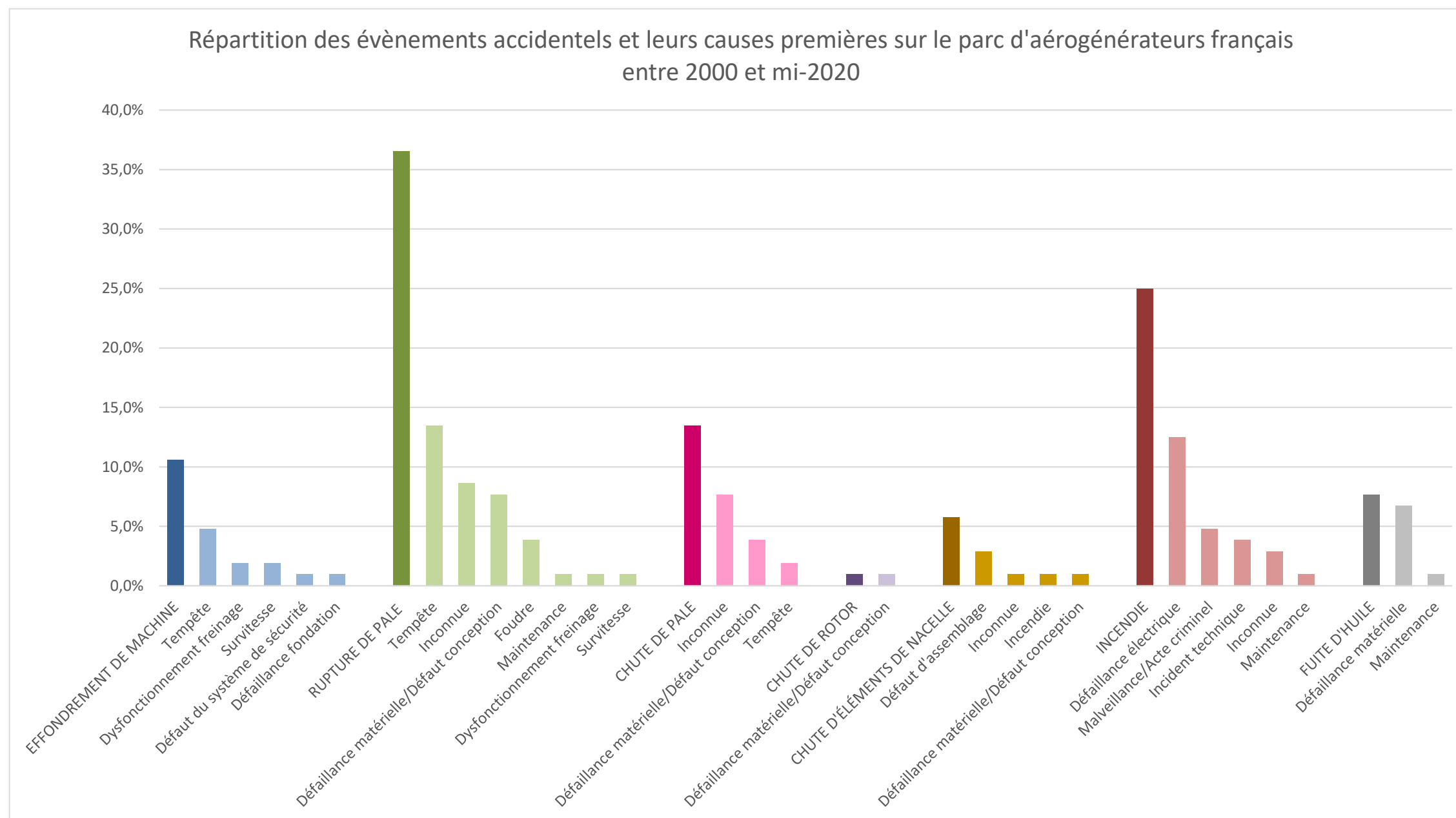
Figure 6 : Répartition des accidents et de leurs causes premières sur le parc éolien français entre 2000 et septembre 2020 (Source : ENCIS Environnement, d'après le Guide technique, mai 2012)
