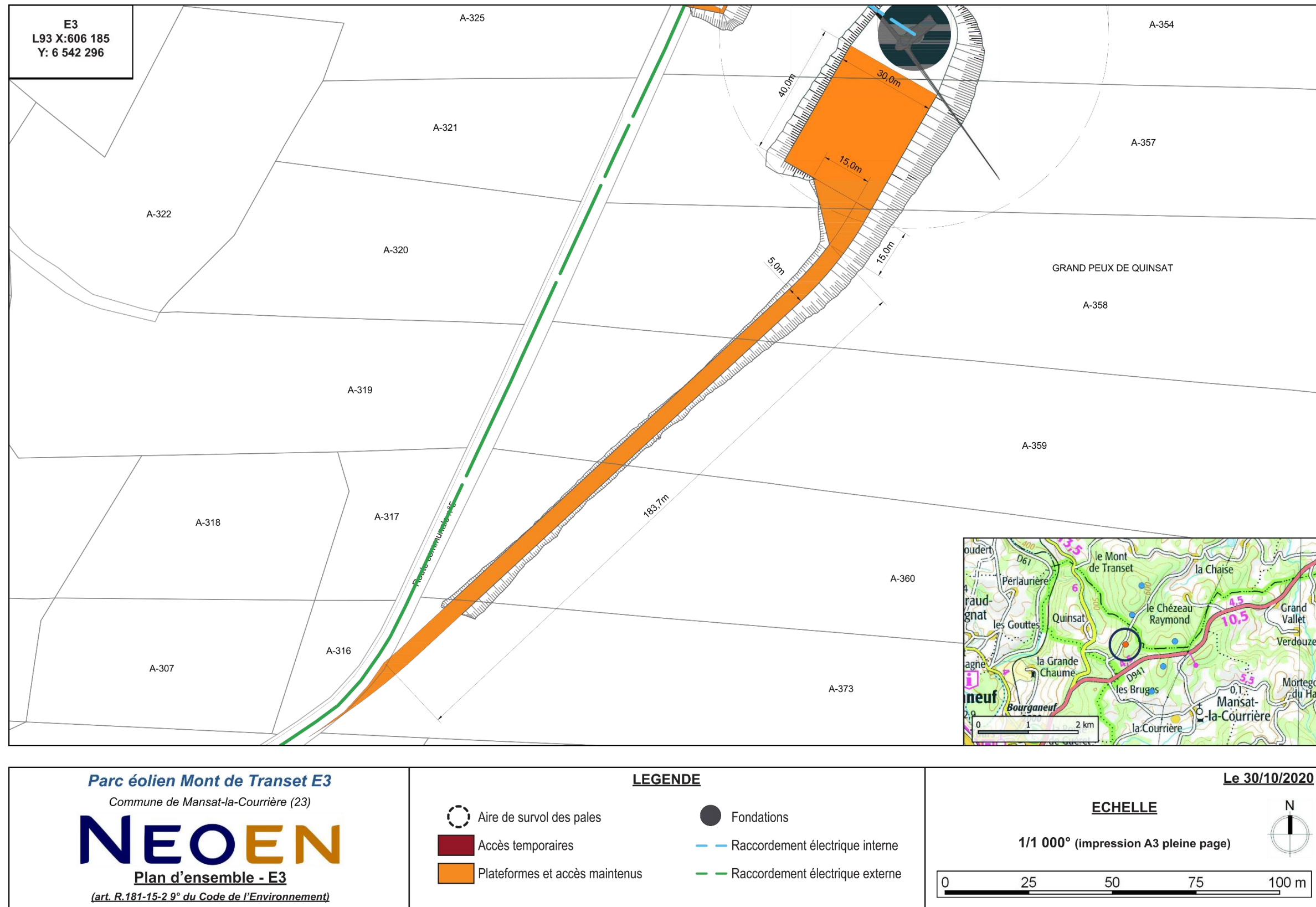
Carte 14 : Plan de masse du parc éolien du Mont de Transet – E3 (2/2)
