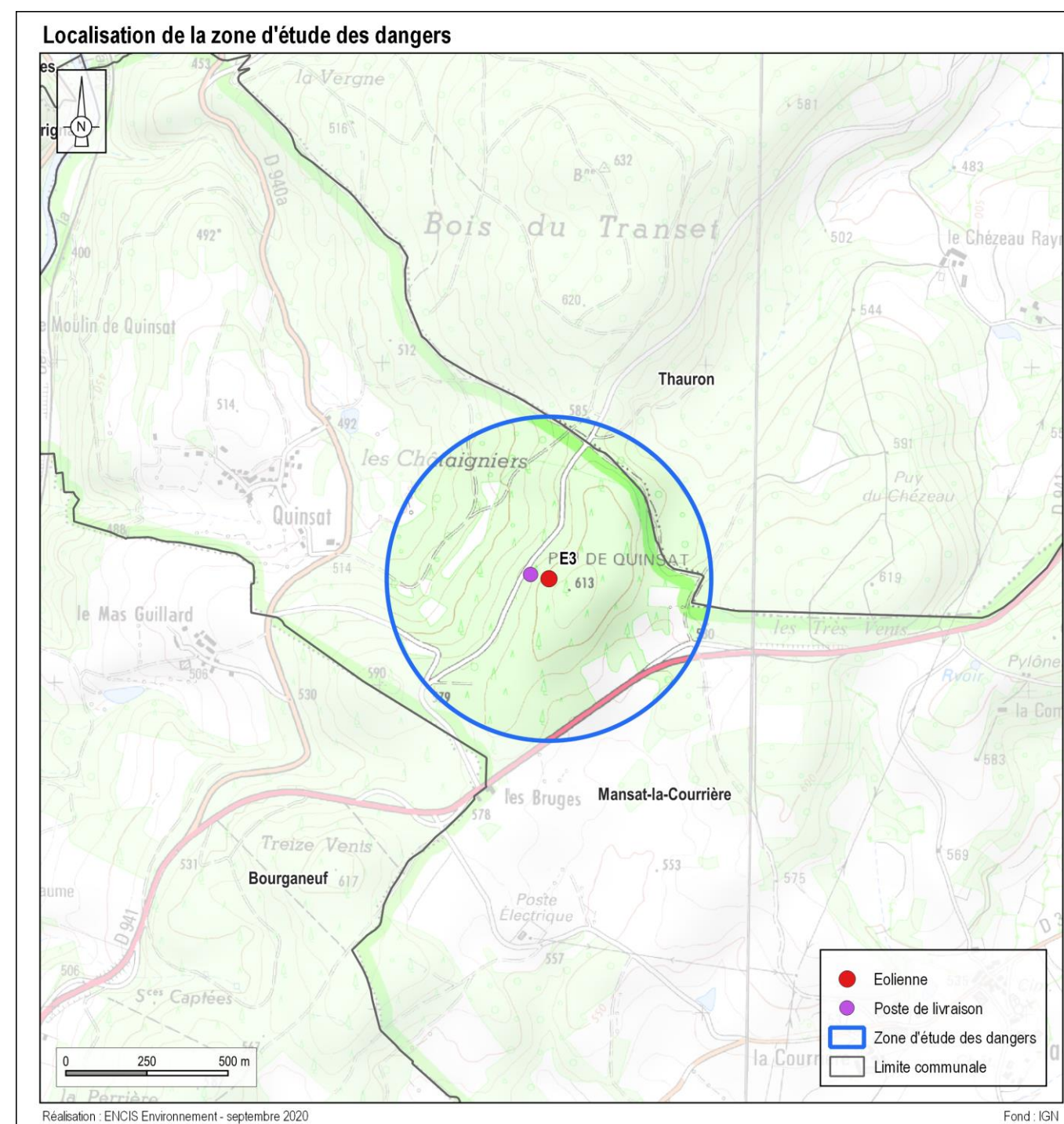
Carte 3 : Zone d'étude et aires d'études des dangers définies autour de l'aérogénérateur
