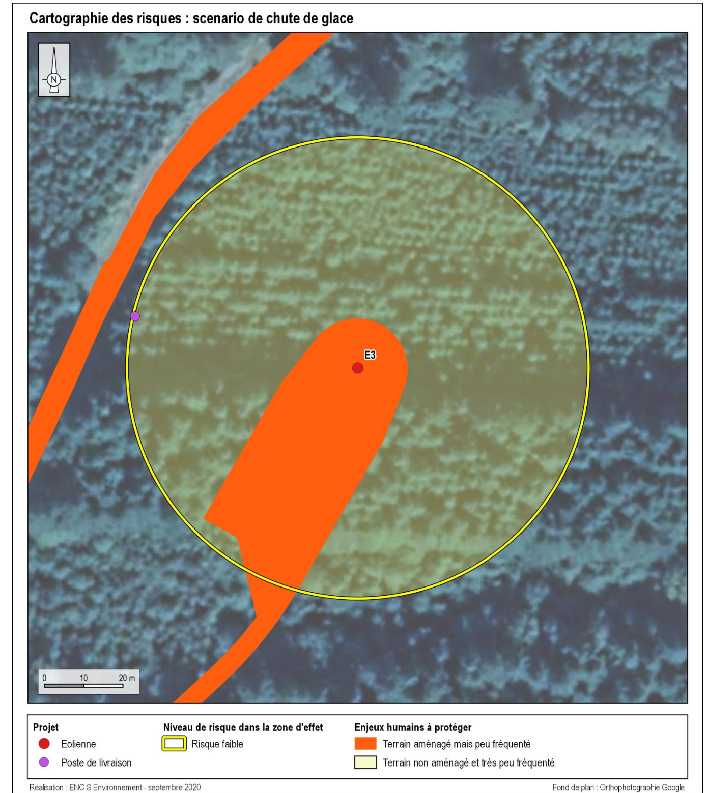
Carte 21 : Cartographie des risques – Scénario de chute de glace
