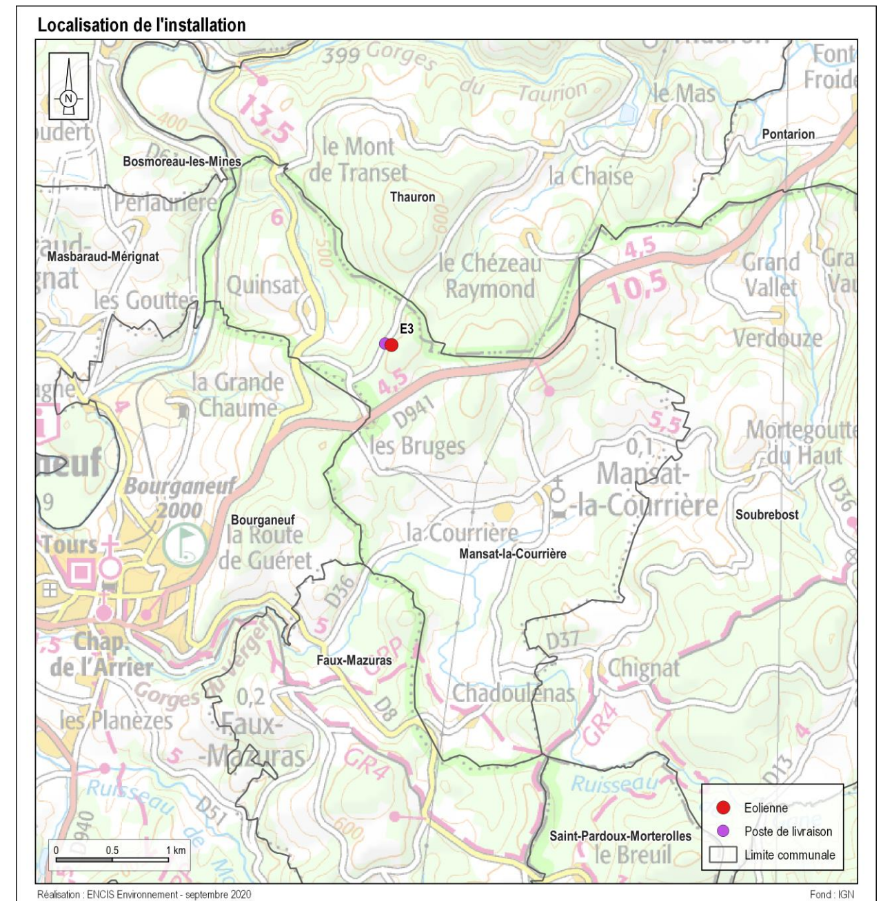
Carte 2 : Localisation de l'éolienne du parc éolien du Mont de Transet - E3
