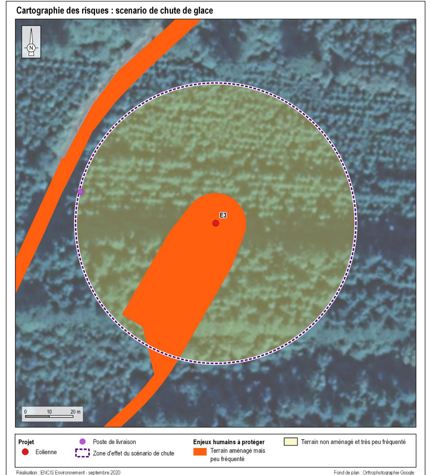
Carte 16 : Cartographie des enjeux identifiés dans les zones d'effet du scénario de chute de glace
