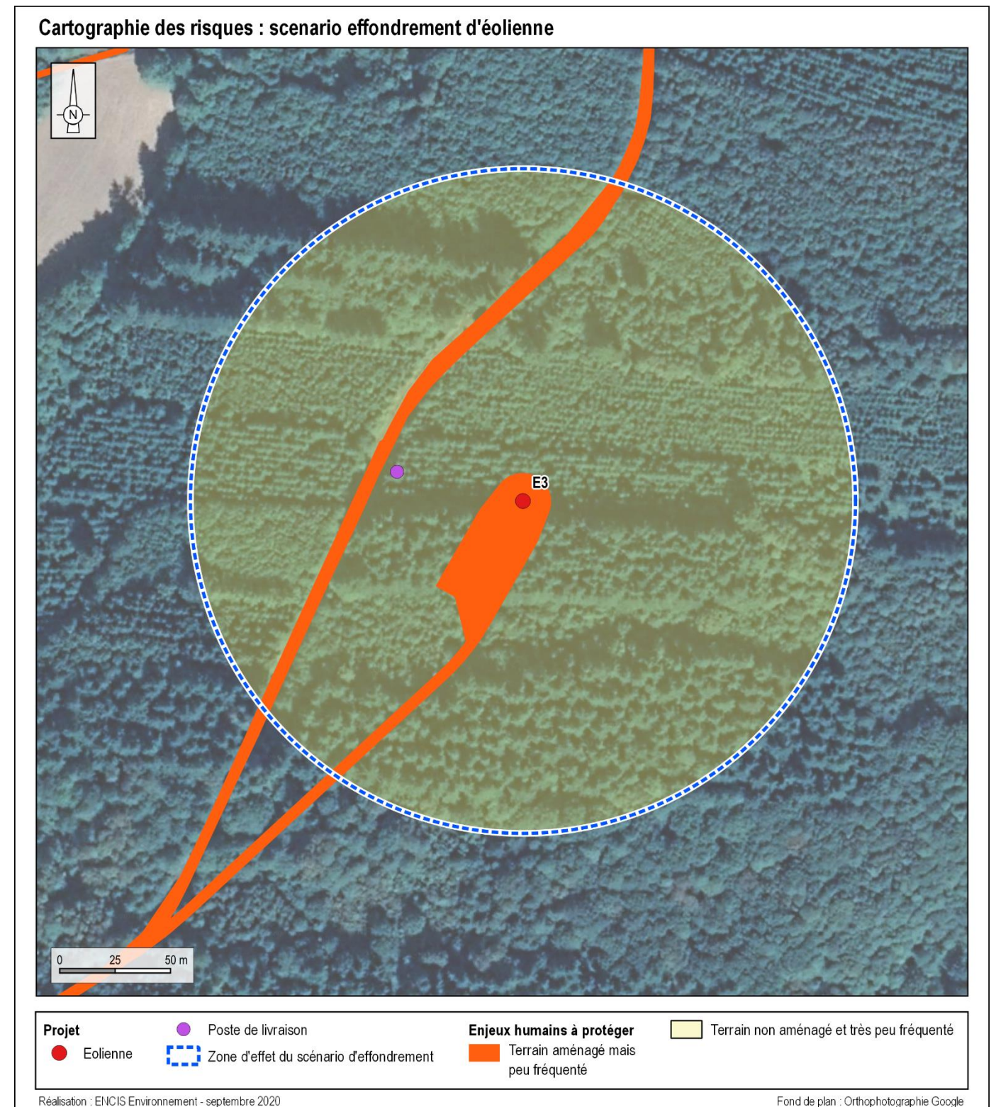
Carte 15 : Cartographie des enjeux identifiés dans la zone d'effet du scénario d'effondrement d'éolienne
