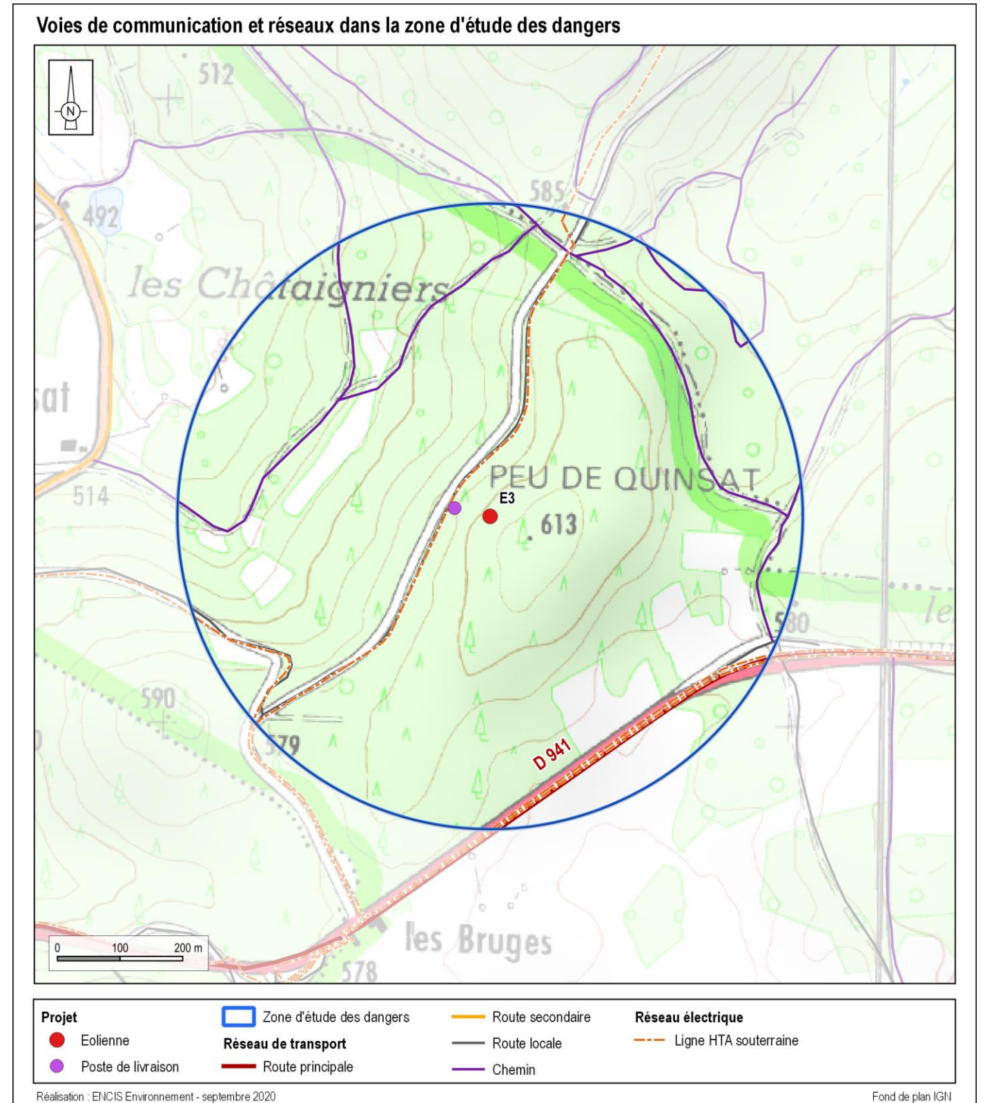
Carte 10 : Voies de communication et réseaux dans la zone d'étude des dangers
